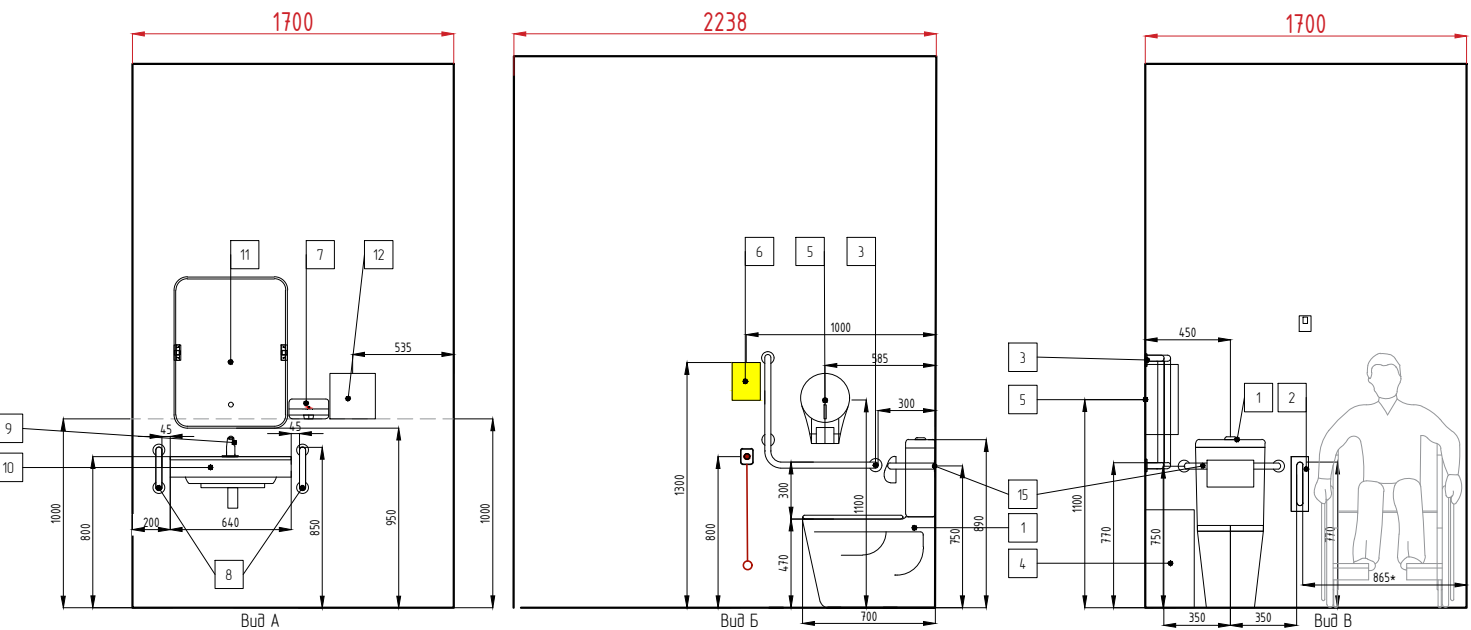
Развертки универсальной кабины уборной 1700x2200 с угловым левым (правым) расположением унитаза
